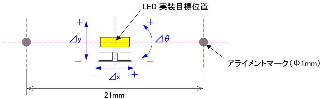
図 9. 実装精度評価方法
