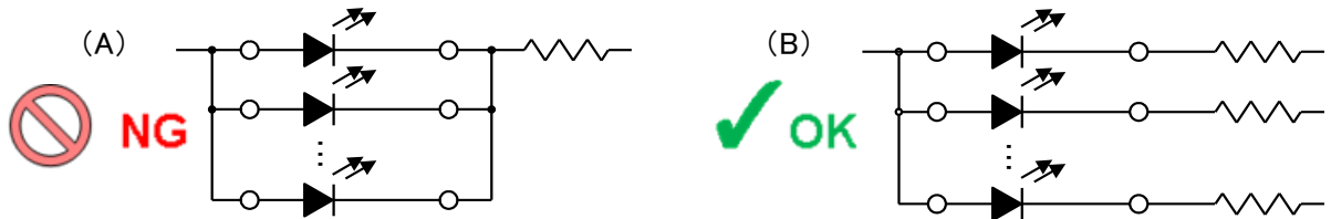
図 2. 並列回路の例
