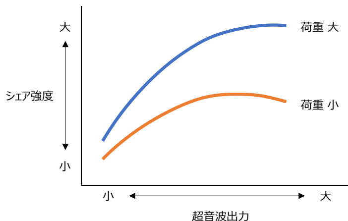
図 6. 超音波出力と荷重の交互作用のイメージ
