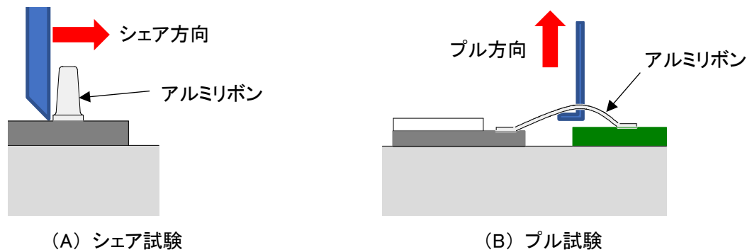
図 5. 接合強度評価方法
