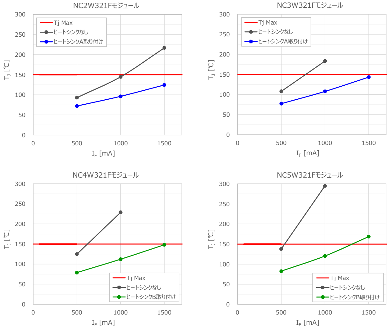
図 8. 駆動電流とジャンクション温度 ( T_A = 50^{\circ}\text{C} )
