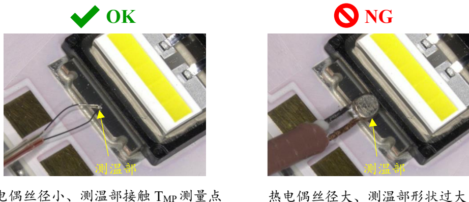
图 2. 热电偶安装例 (热电偶丝焊接前)
