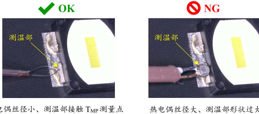
图 2. 热电偶安装例 (热电偶丝焊接前)
