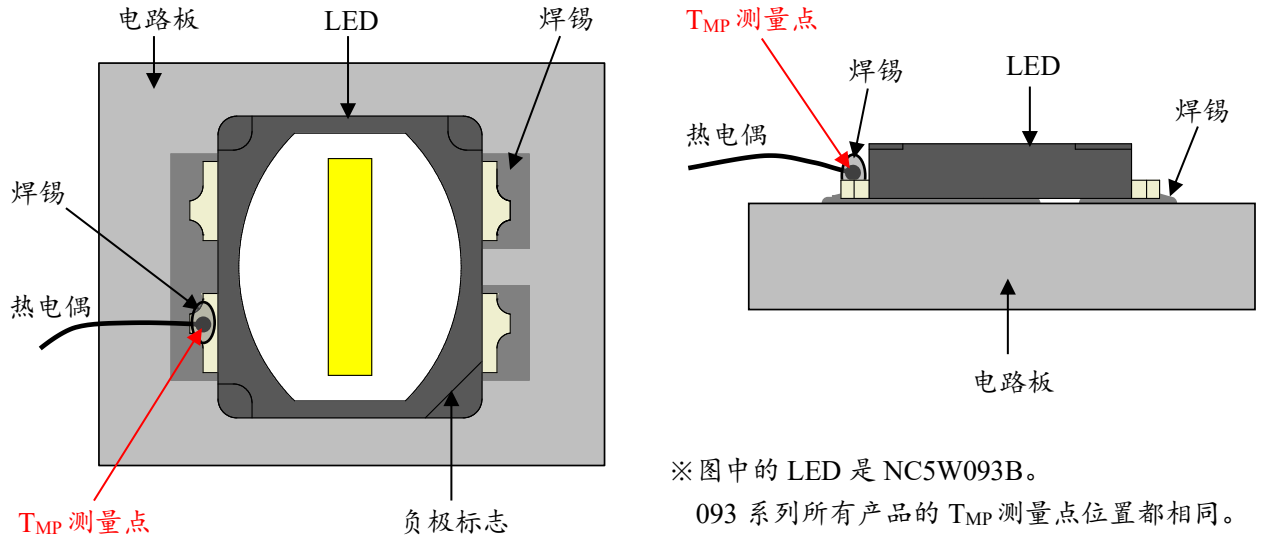
图 1. T MP 测量点
