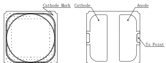
図3 T_s 測定ポイント (NVSU233C-D4)
