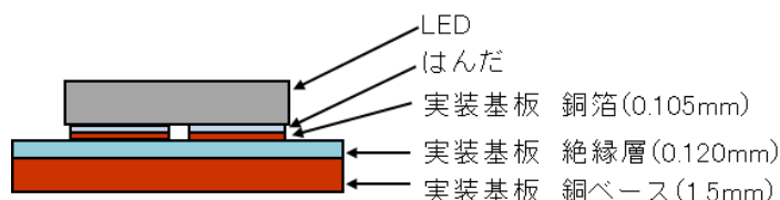
図 4 実装構造
