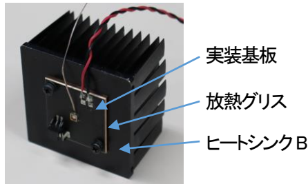
写真 4 評価した光源の構成 (NVSU233C)
