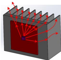
図 5 フィンを垂直に設置したときの 熱経路イメージ図
