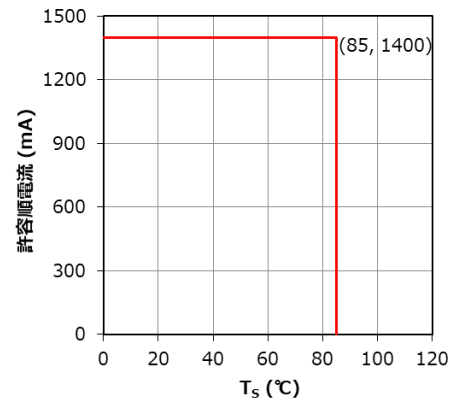
図1 T_s - 許容順電流特性
