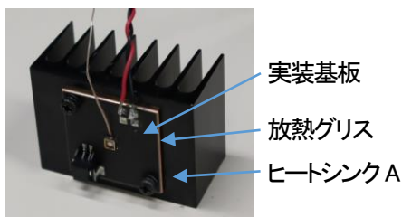
写真 3 評価した光源の構成 (NVSU233C)
