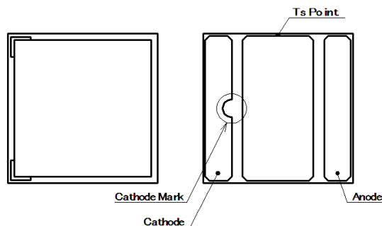
図2 T_S 測定ポイント
