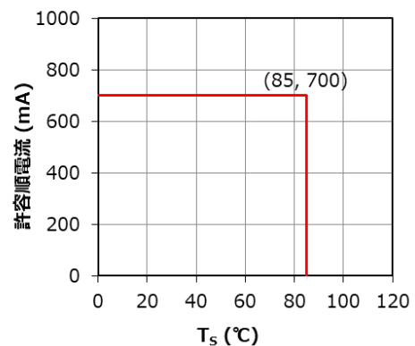
図1 T_S - 許容順電流特性
