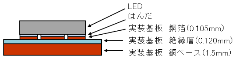
図3 実装構造
