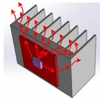
図4 フィンを垂直に設置したときの 熱経路イメージ図
