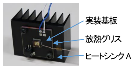
写真2 評価した光源の構成
