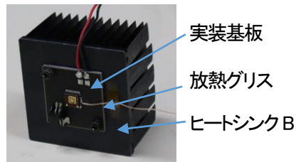
写真3 評価した光源の構成
