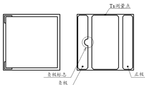
图 2 T_S 测量点
