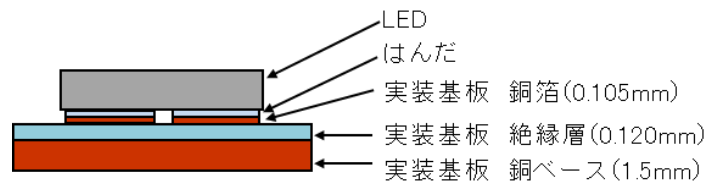
図3 実装構造
