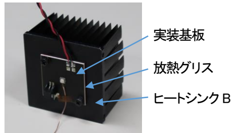
写真3 評価した光源の構成
