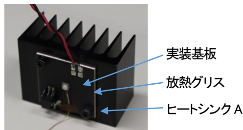
写真2 評価した光源の構成
