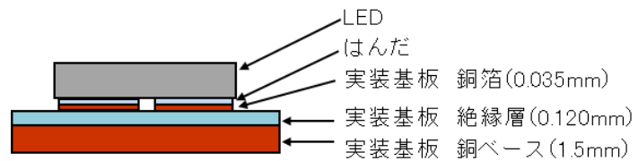
図5 実装構造
