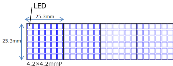
図7 光源 (実装基板1枚にLEDを6×6pcs.搭載×4枚)
