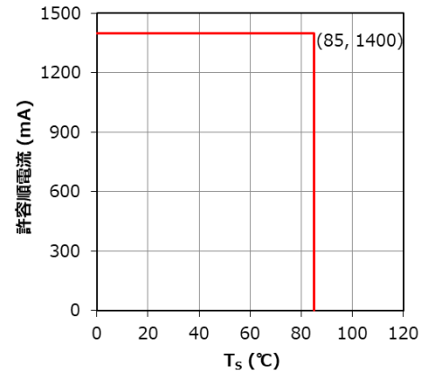
図1 T_S - 許容順電流特性
