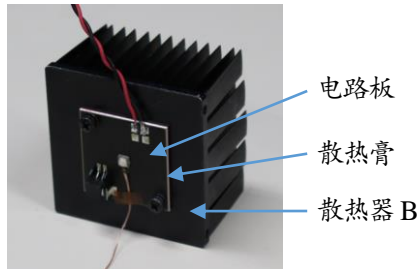
照片 3 评价光源的散热结构
