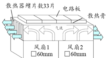
图 6 评价光源的散热结构
