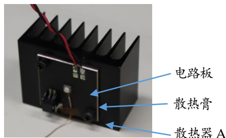
照片 2 评价光源的散热结构
