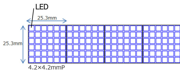
图 7 光源 (安装有 6\times 6 粒LED的电路板4块)
