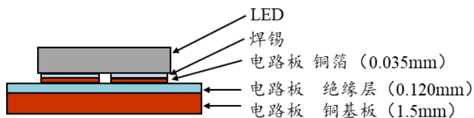
图 5 电路板安装时结构
