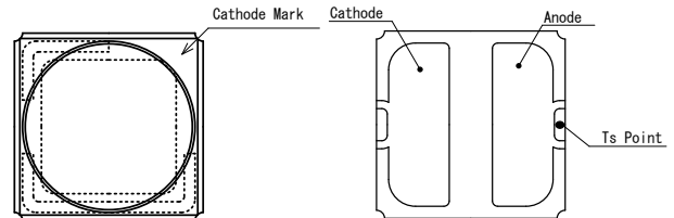
図3 T_S 測定ポイント (NVSU233B-D4)
