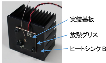
写真4 評価した光源の構成 (NVSU233B)
