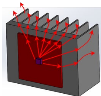
図5 フィンを垂直に設置したときの 熱経路イメージ図
