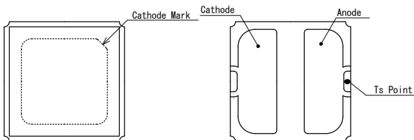
図2 T_S 測定ポイント (NVSU233B)
