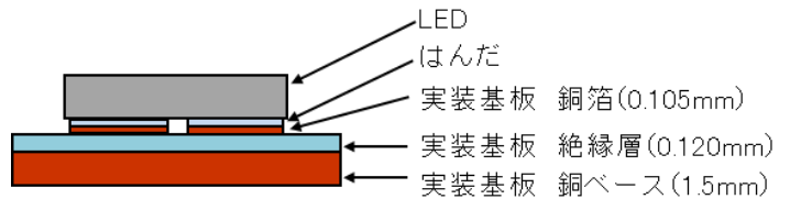
図 4 実装構造
