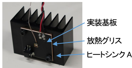
写真 3 評価した光源の構成 (NVSU233B)
