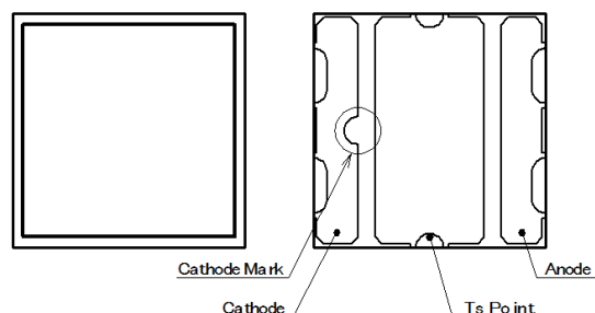
図2 T_S 測定ポイント
