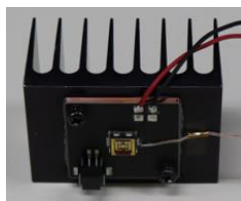
写真4 フィン垂直 (弊社設置の向き)
