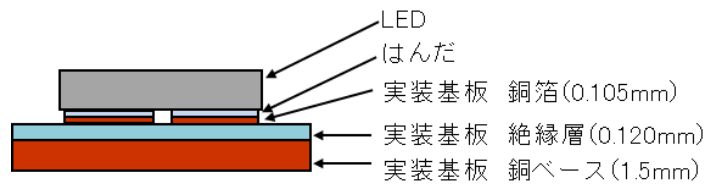
図3 実装構造
