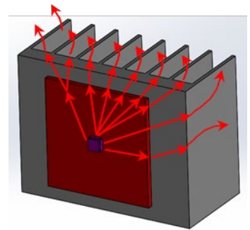
图 4 让鳍片向侧面设置时的 散热路径示意图
