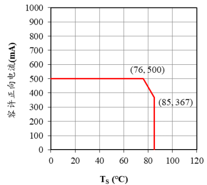
图 1 “ T_S vs. 容许正向电流”特性
