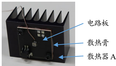
照片 2 评价光源的散热结构
