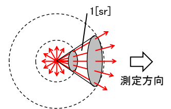
図 5. 光度の定義
