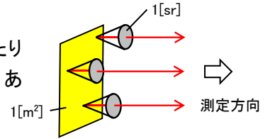
図 10. 輝度の定義
