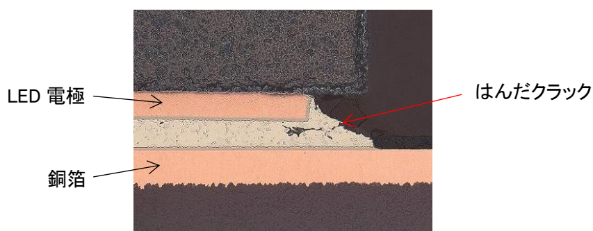
図1. はんだクラックの発生例
