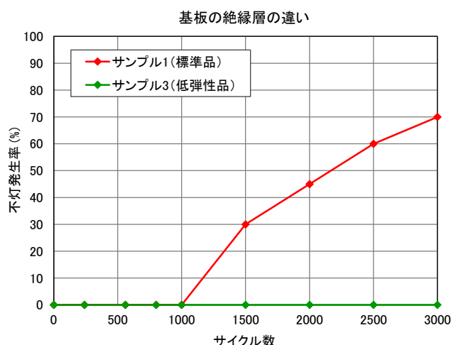
図 10. 不灯発生率および \Delta V_F 平均値
