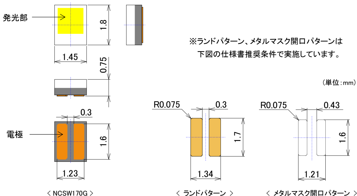
図 8. 各種図面
