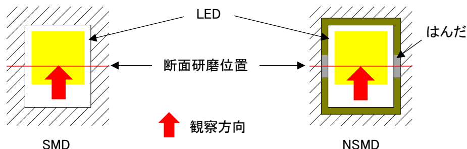
図 12. 断面研磨位置および観察方向
