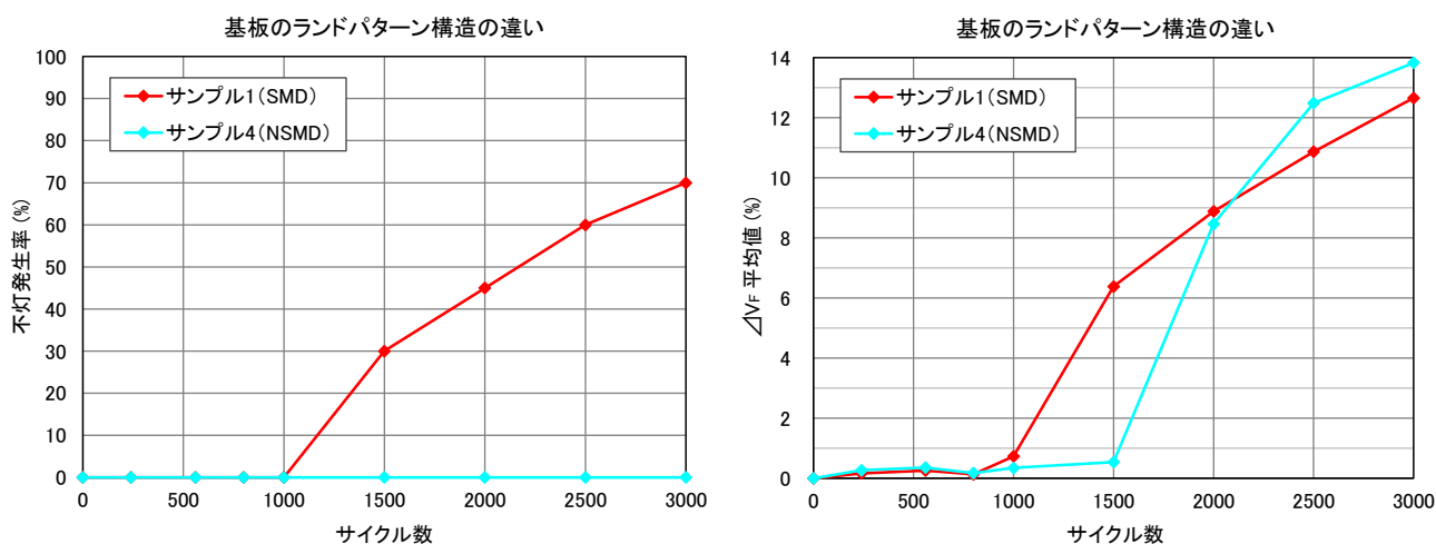
図 11. 不灯発生率および \Delta V_F 平均値
