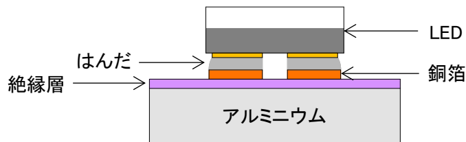
図 2. LED 実装状態
