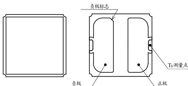
图 2 T_S 测量点
