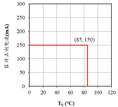
图 1 “ T_S vs. 容许正向电流”特性
