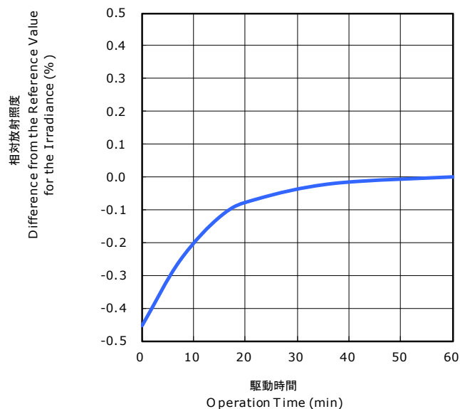
駆動時間 vs 放射照度 Operation Time vs Irradiance
