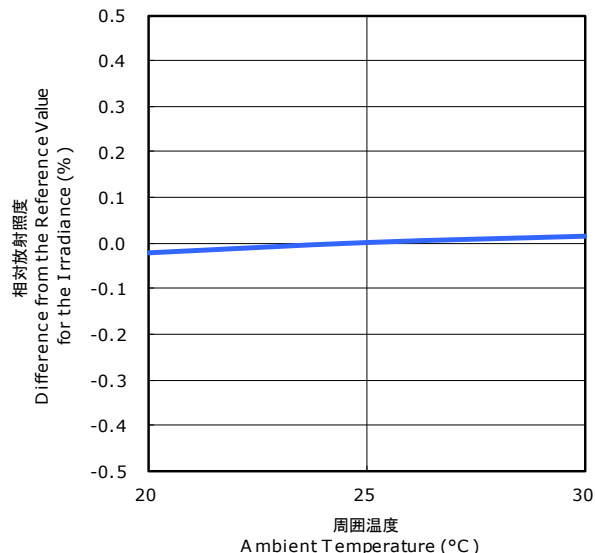
周囲温度 vs 放射照度 Ambient Temperature vs Irradiance
