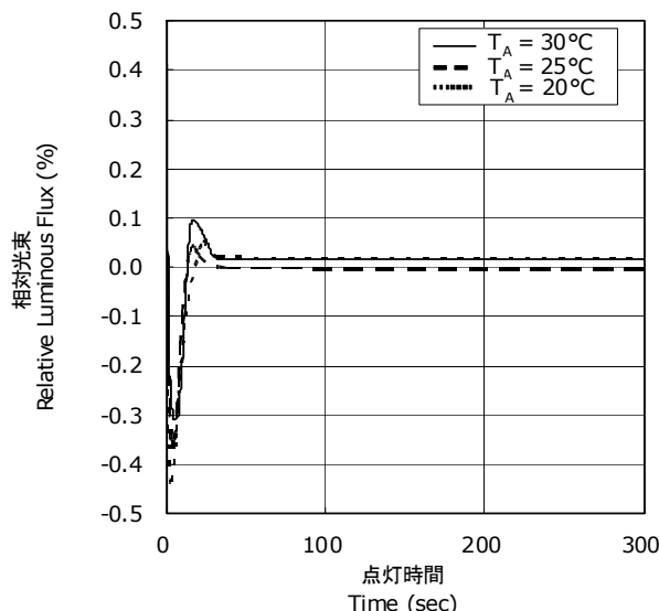
点灯時間 - 相对光束特性 Relative Luminous Flux Over Time
