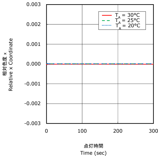
点灯時間 - 相对色度 x特性 Relative x Coordinate Over Time
