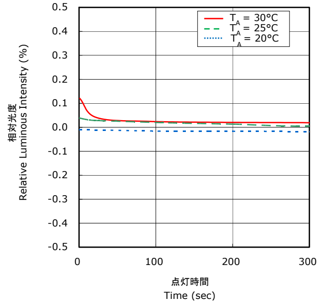
点灯時間 - 相对光度 Relative Luminous Intensity Over Time
