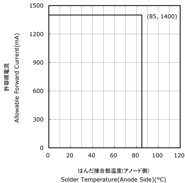
はんだ接合部温度(アノード側)-許容順電流特性 Solder Temperature (Anode Side) vs Allowable Forward Current
