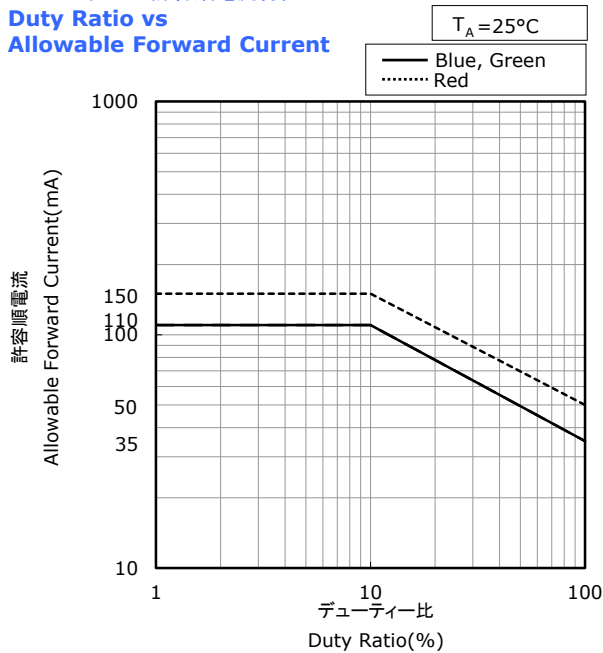
デューティ比-許容順電流特性
