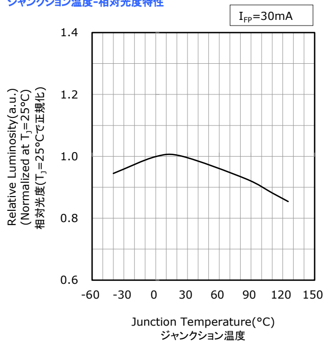
Junction Temperature vs Relative Luminosity ジャンクション温度-相対光度特性
