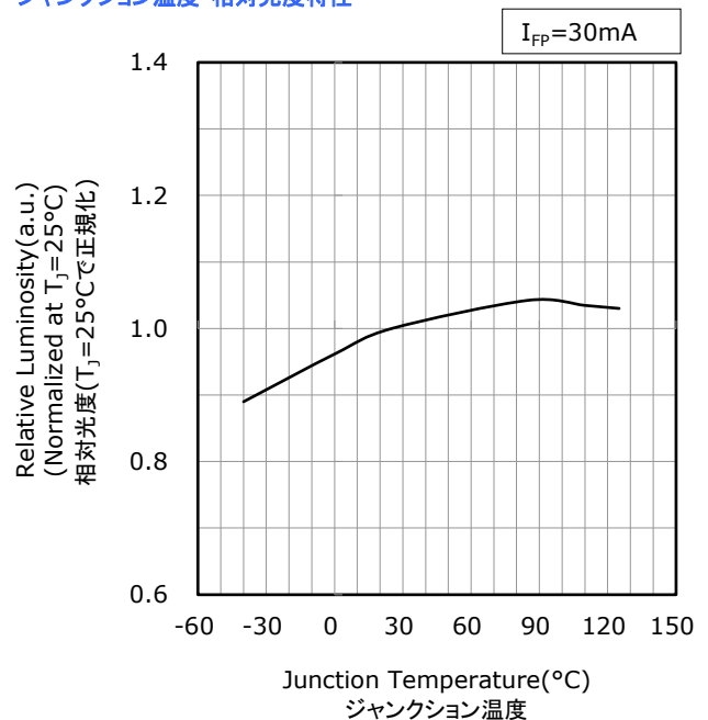
Junction Temperature vs Relative Luminosity ジャンクション温度-相対光度特性
