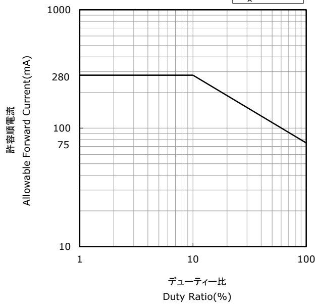
デューティ比-許容順電流特性 Duty Ratio vs Allowable Forward Current
