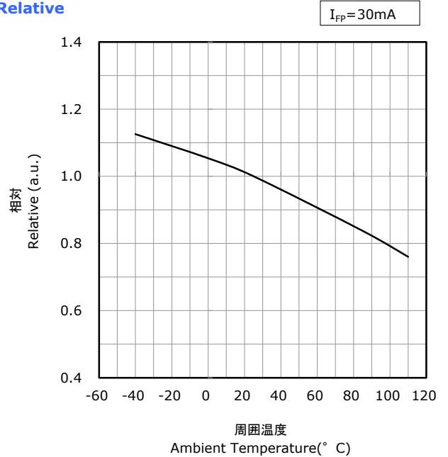
周囲温度-相対 特性 Ambient Temperature vs Relative
