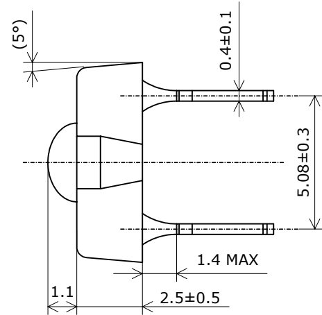
ストッパー部詳細図 Lead Standoff
