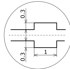
ストッパー部詳細図 Lead Standoff
