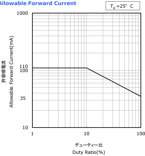
デューティ比-許容順電流特性 Duty Ratio vs Allowable Forward Current
