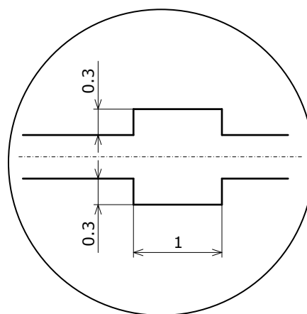
ストップパー部詳細図 Lead Standoff
