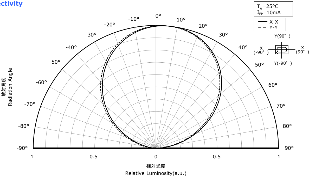
指向特性 Directivity
