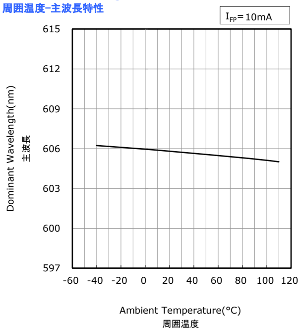
Ambient Temperature vs Dominant Wavelength 周囲温度-主波長特性
