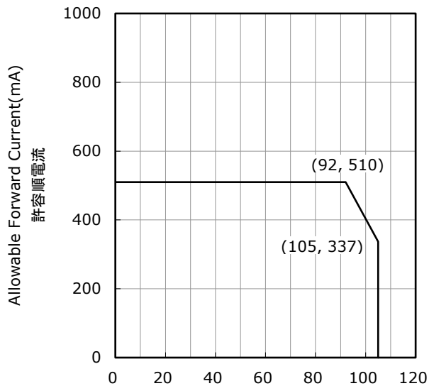
Temperature at Measurement Point on a Case(°C) ケース温度測定部温度
