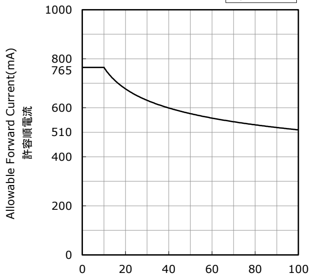
Duty Ratio(%) デューティー比
