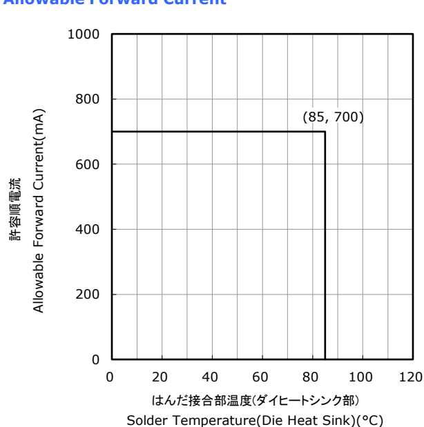
はんだ接合部温度(ダイヒートシンク部)-許容順電流特性
